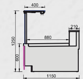
REFRIGERAZIONE VENTILATA VENTILATED REFRIGERATION RÉFRIGÉRATION VENTILÉE
