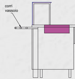
PIANO FREDDO VENTILATO INSERIMENTO PER MODULI L.100 / 125 / 150cm
