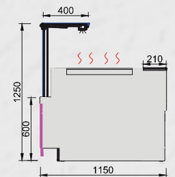
CALDO SECCO DRY HEAT CHALEUR SÈCHE
