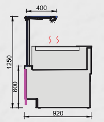
CALDO SECCO DRY HEAT CHALEUR SÈCHE
