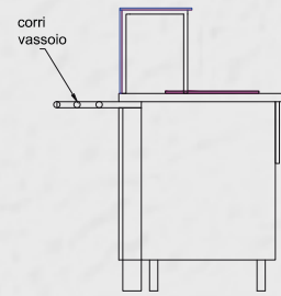
PIANO FREDDO A CONTATTO INSERIMENTO PER MODULI L.100 / 125 / 150cm
