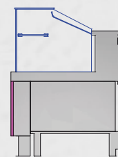
VETRINA CALDO SECCO VETRI BASSI DIRITTI L.100 / 125 / 150cm
