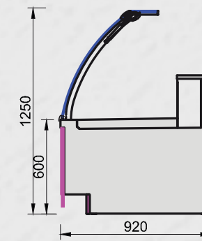
REFRIGERAZIONE STATICA STATIC REFRIGERATION RÉFRIGÉRATION STATIQUE
