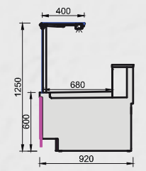
REFRIGERAZIONE STATICA STATIC REFRIGERATION RÉFRIGÉRATION STATIQUE
