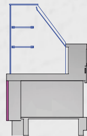
VETRINA FREDDO VENTILATO VETRI ALTI DIRITTI L.100 / 125 / 150cm
