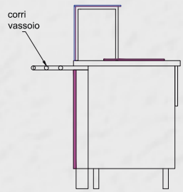
PIANO CALDO SECCO INSERIMENTO PER MODULI L.100 / 125 / 150cm
