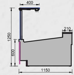
REFRIGERAZIONE CON SERPENTINA A CONTATTO PER PESCE REFRIGERATION WITH COIL TO CONTACT FOR FISH RÉFRIGÉRATION AVEC SERPENTINE AU CONTACT POUR POISSON
