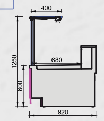
REFRIGERAZIONE VENTILATA VENTILATED REFRIGERATION RÉFRIGÉRATION VENTILÉE
