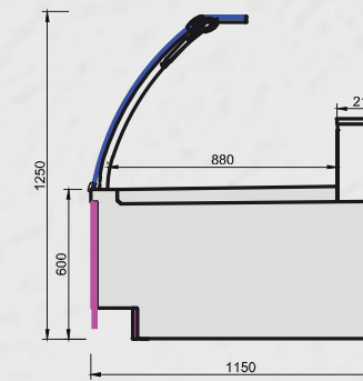
REFRIGERAZIONE VENTILATA VENTILATED REFRIGERATION RÉFRIGÉRATION VENTILÉE
