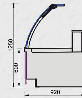
REFRIGERAZIONE VENTILATA VENTILATED REFRIGERATION RÉFRIGÉRATION VENTILÉE
